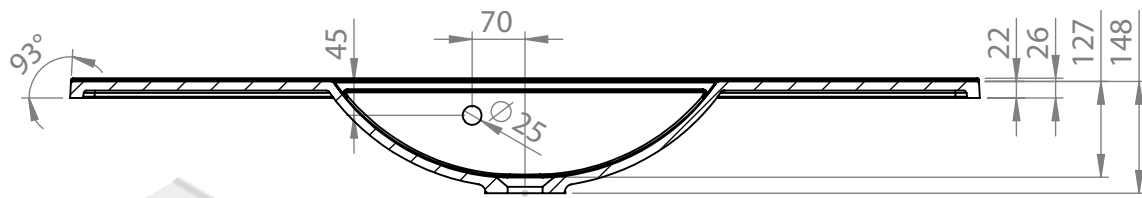
PRZEKRÓJ H-H
